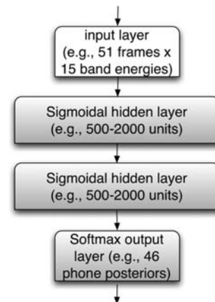
Fig. 5. 15 \times 51 MLP4.
